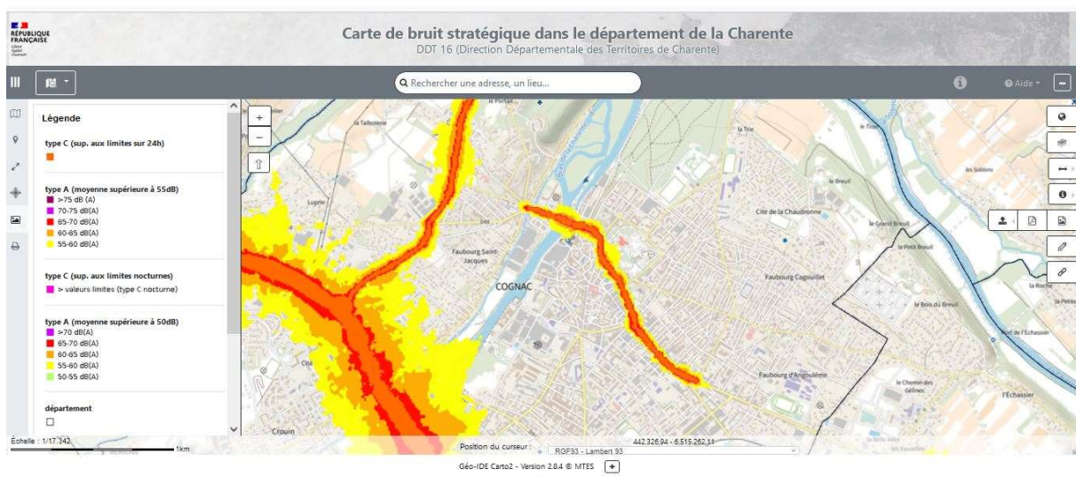
Extrait de la Carte de Bruit Stratégique
